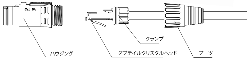
● SE8FC-LOD-C6A (パーツ詳細図)
