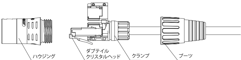
● SE8MC-02-30-LOD (パーツ詳細図)
