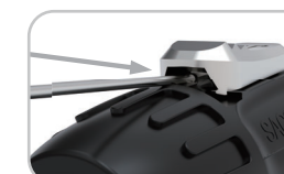
ラッチキー後部底面のボタンを 小型工具で前方に押して操作
