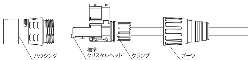
● SE8MC-02-NEW (パーツ詳細図)
