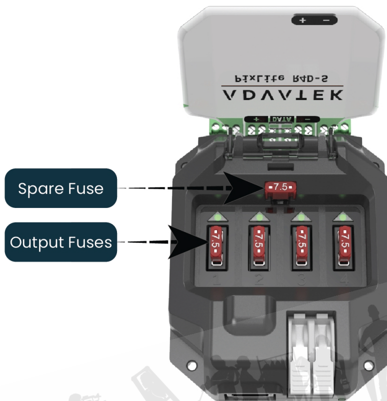
図 6 : PixLite R4D-S の内部図
