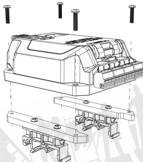
図2：ブラケットに組み付けたレシーバー
