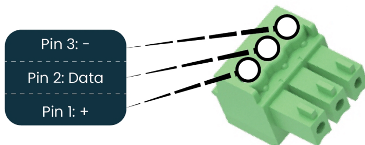
図 9：ピクセル出力ピン配置
