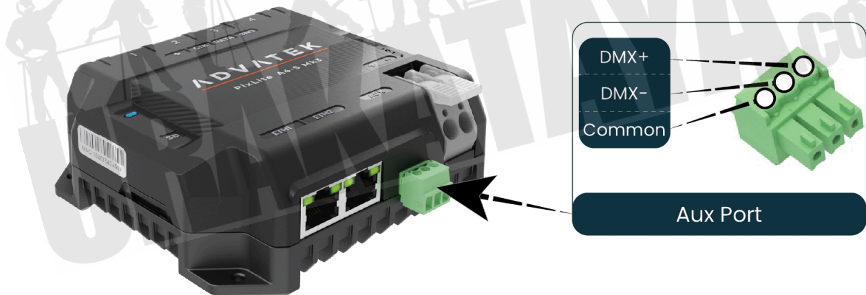
図 13：補助 (AUX) ポートの位置とピン配置
