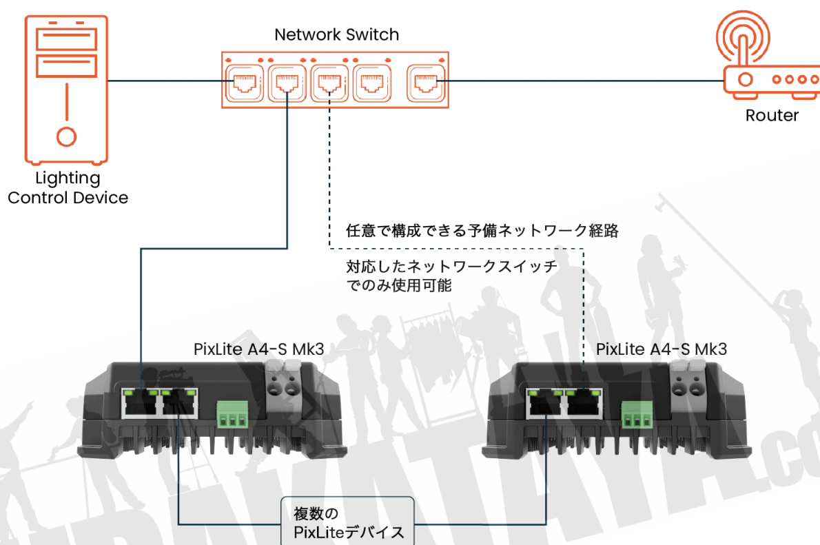
図 14：スイッチとルーターを使用したネットワーク構成例
