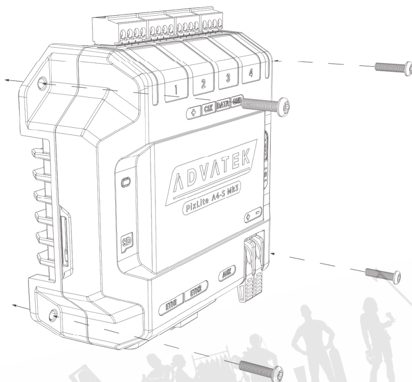
図 2：PixLite A4-S Mk3本体を壁に取り付ける際の位置
