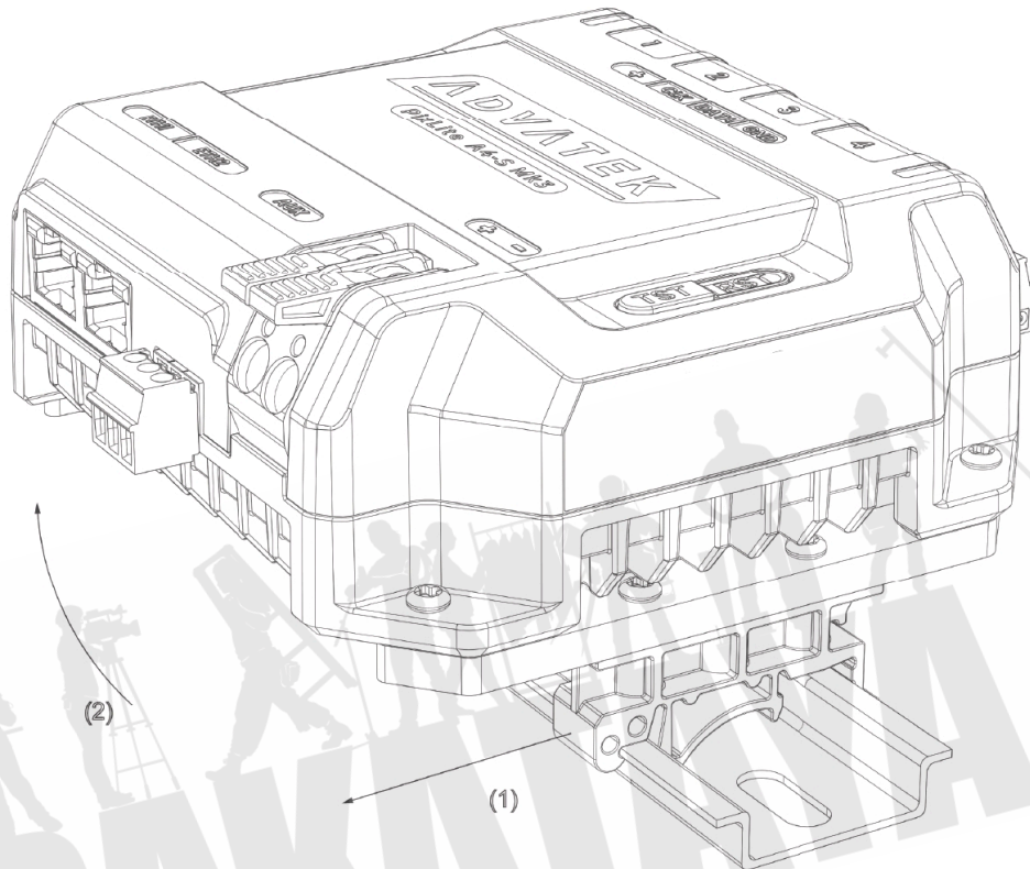
図 5：DINレールから取り外す手順
