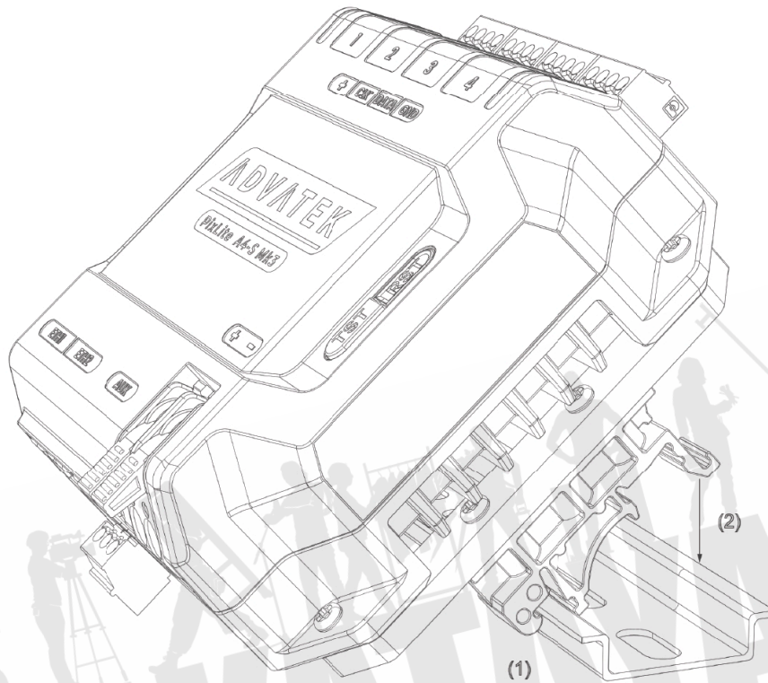
図 4 : DINレールへの取り付け方
